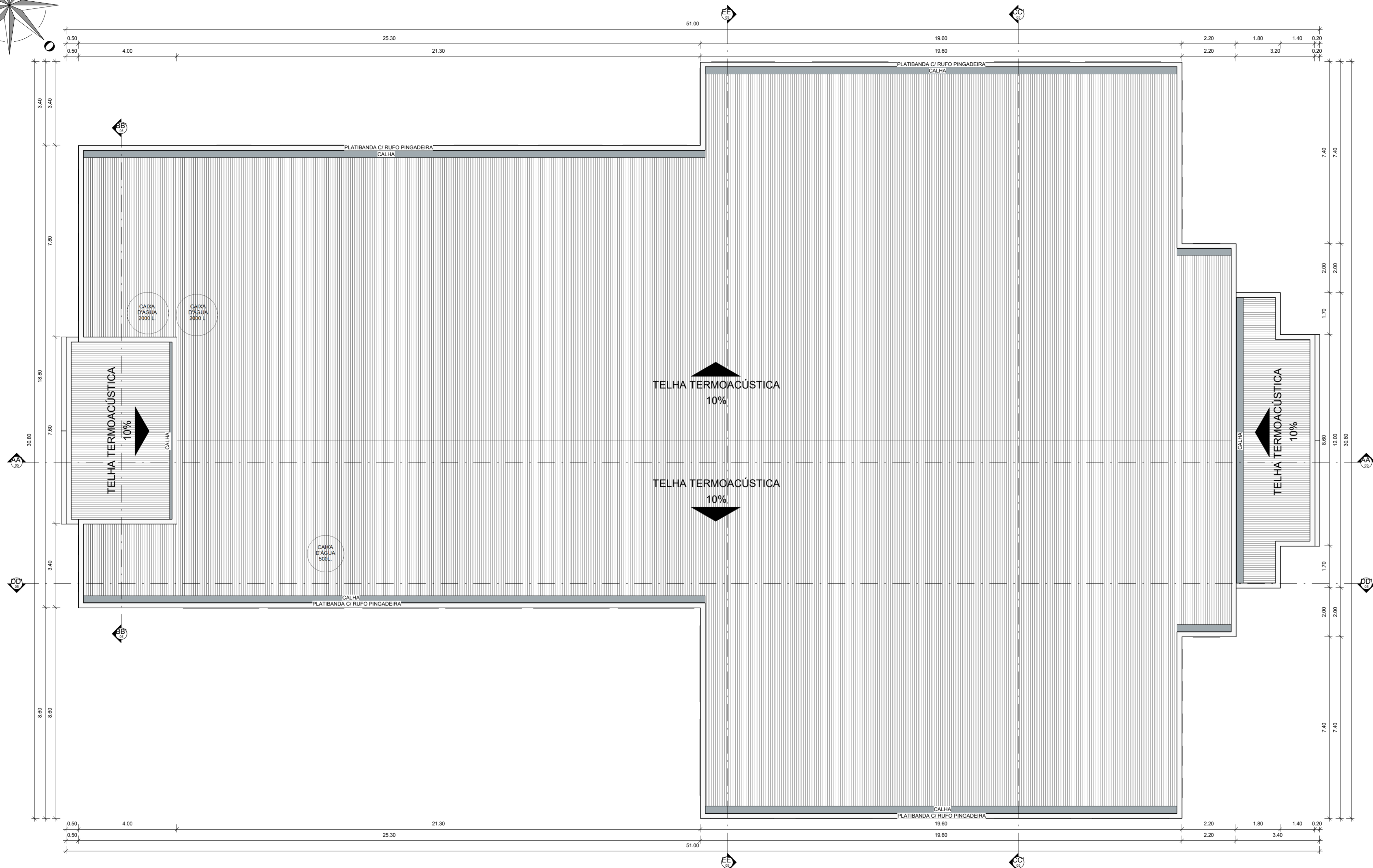
I PLANTA DE COBERTURA 1:100
