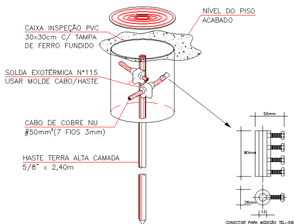
Figura 5 – Haste de aterramento 5/8" com caixa de inspeção Ø 30cm com conexão exotérmica e conector de medição com 4 parafusos
