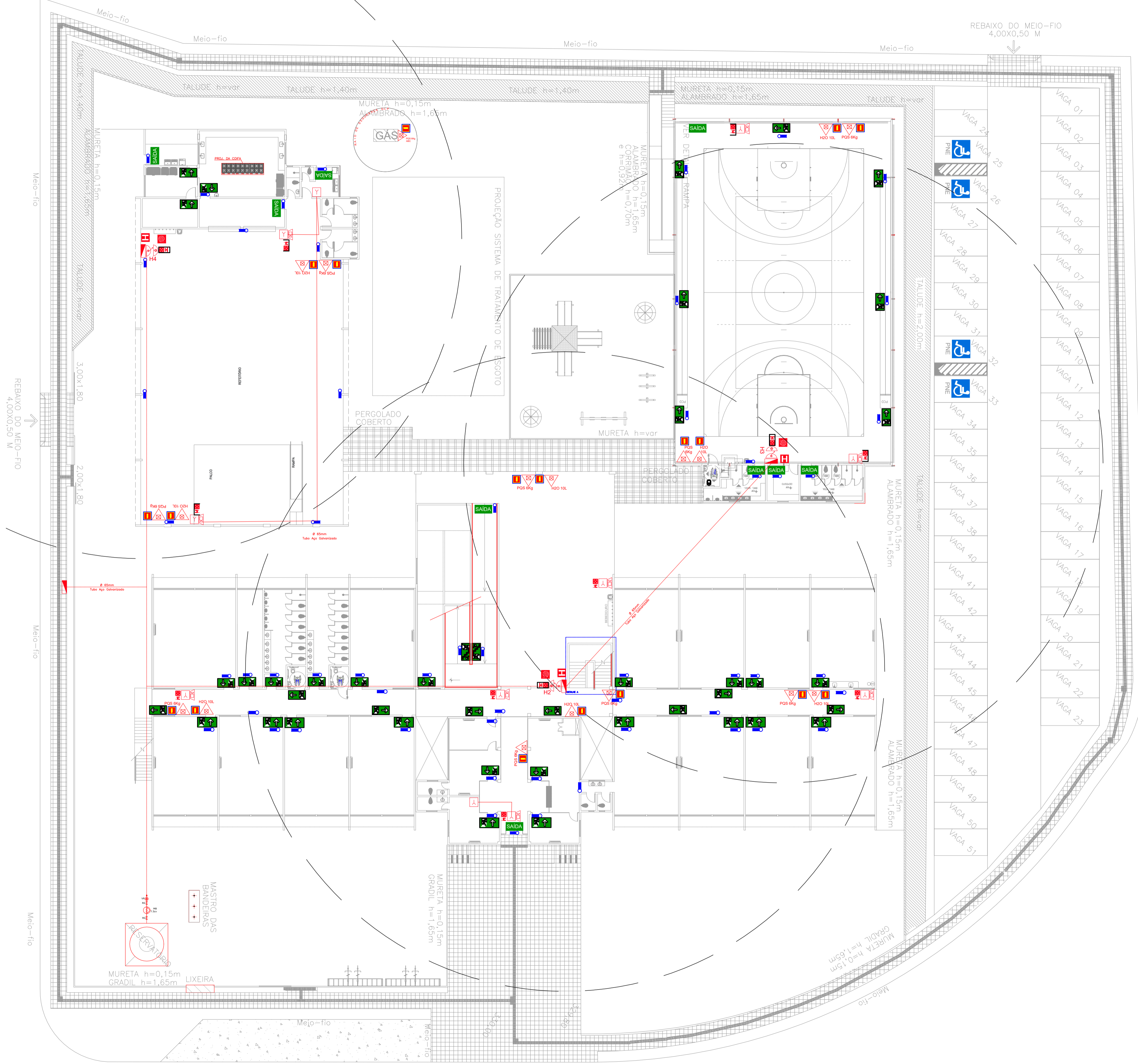
Planta Baixa - Pav. Térreo Esc.: 1/200
