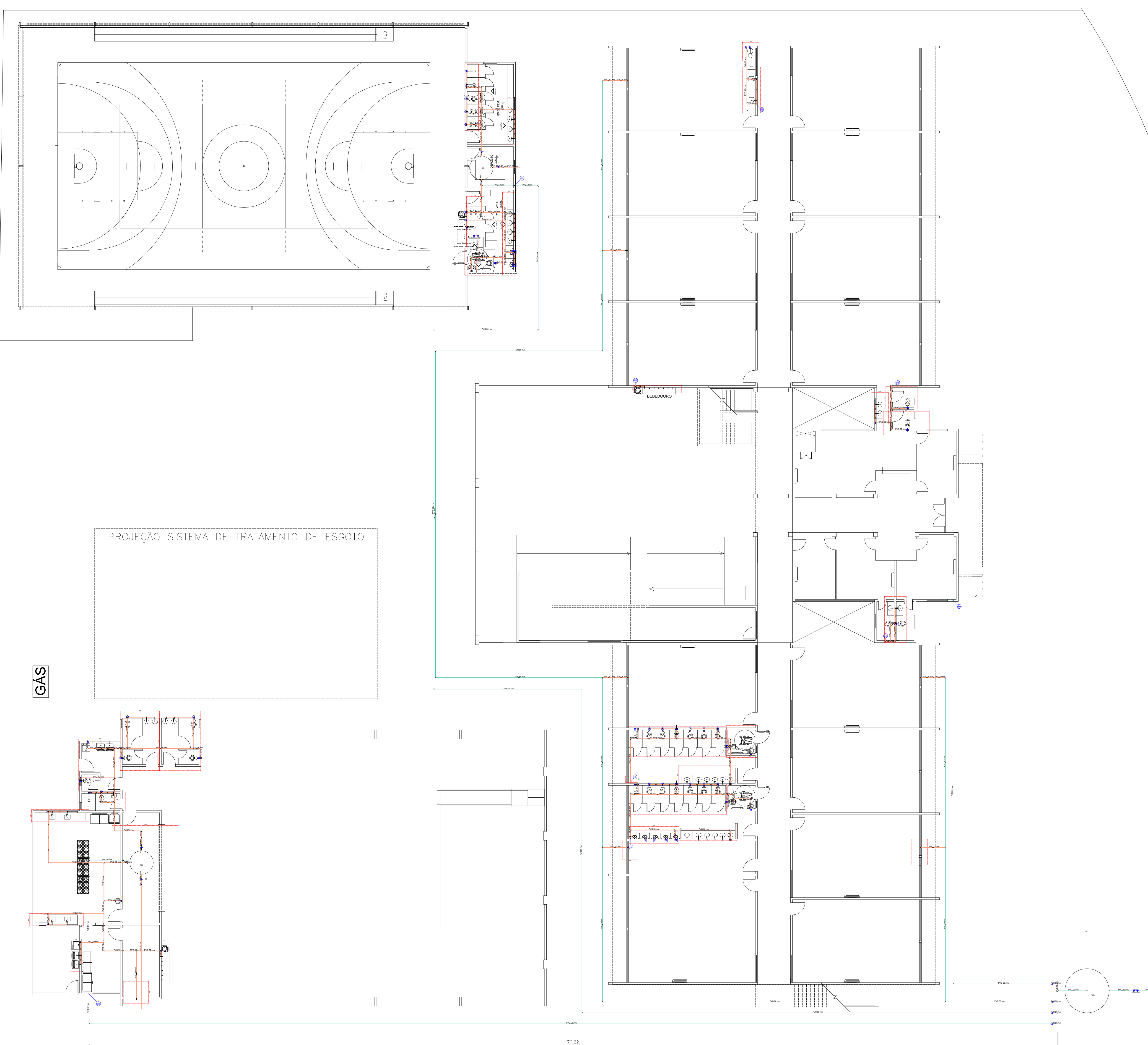
HIDRÁULICO TÉRREO Escala 1:125
