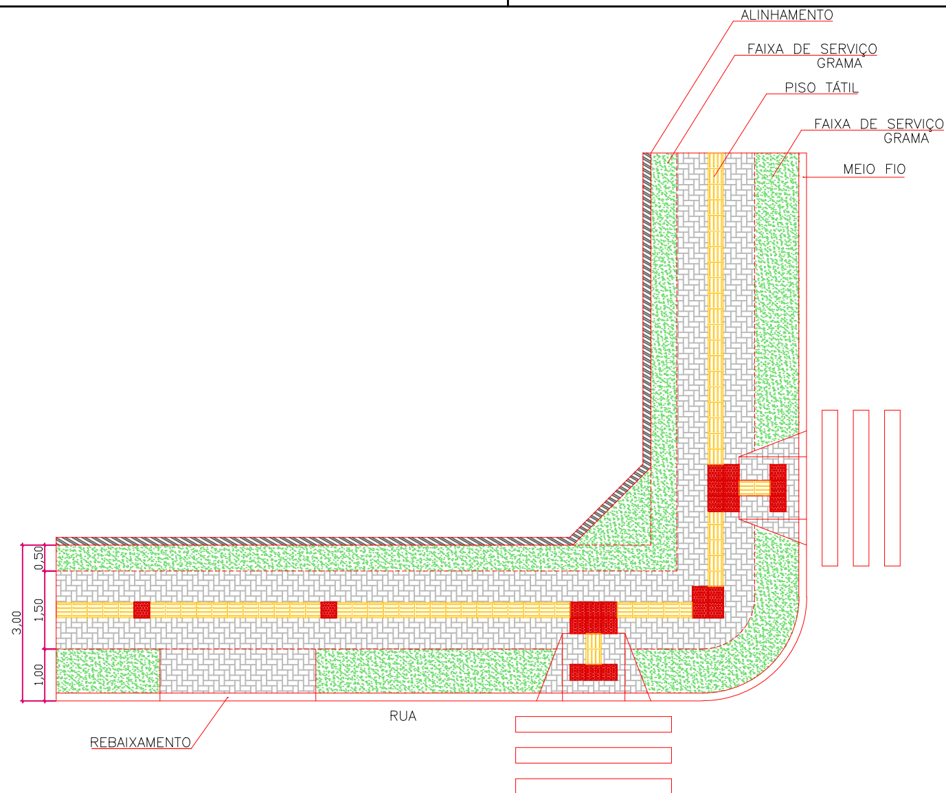
DETALHE - CALÇADA PADRÃO - 3m Sem Escala
