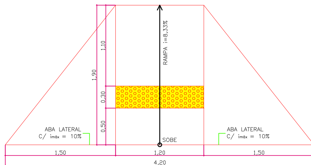
DETALHE - RAMPA DE ACESSO PARA PEDESTRES Sem Escala
