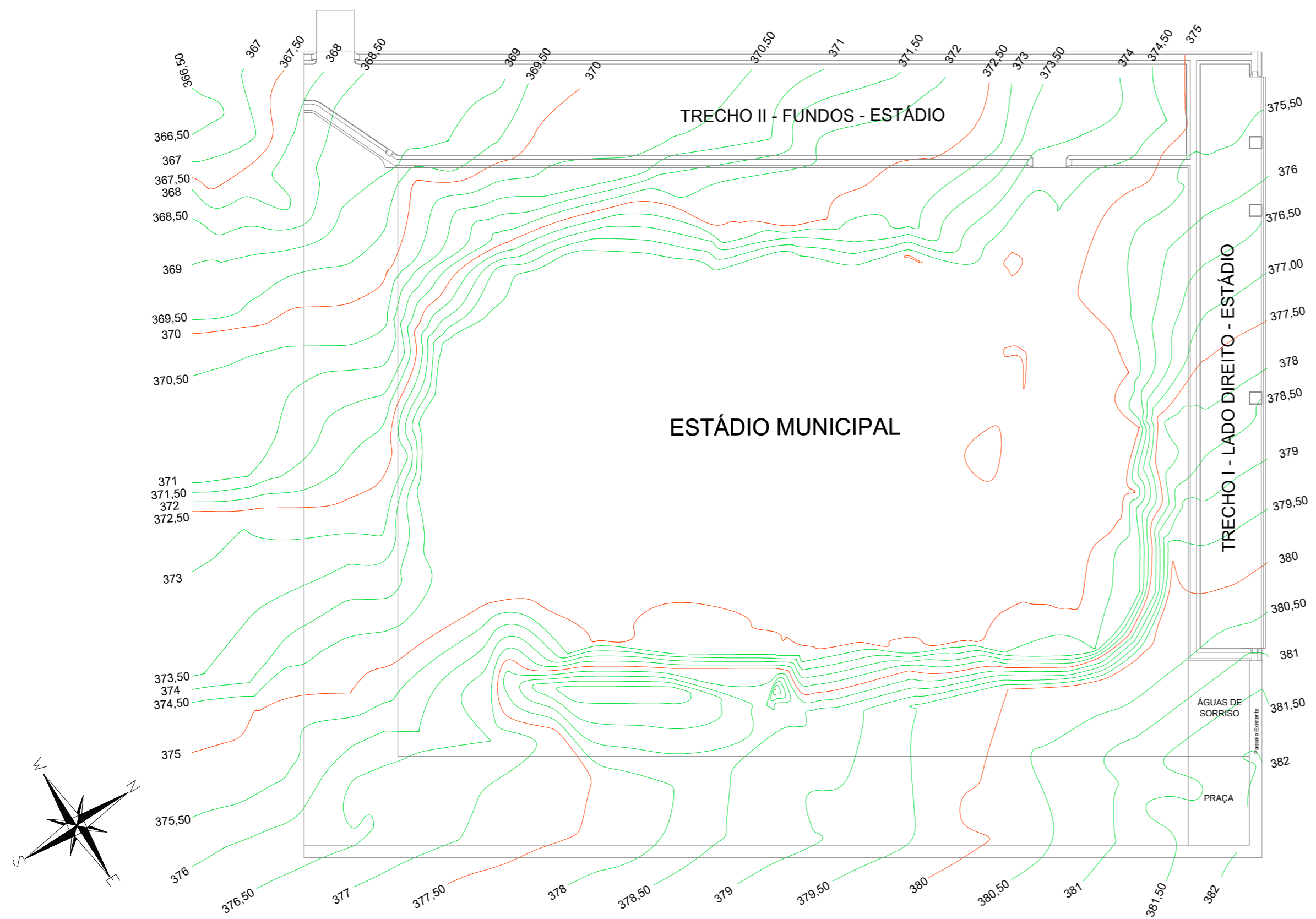
CURVAS DE NÍVEL Escala: 1/100
