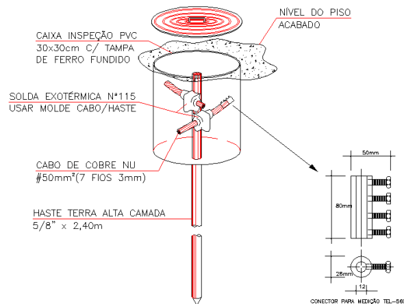
Figura 5 – Haste de aterramento 5/8” com caixa de inspeção Ø 30cm com conexão exotérmica e conector de medição com 4 parafusos
