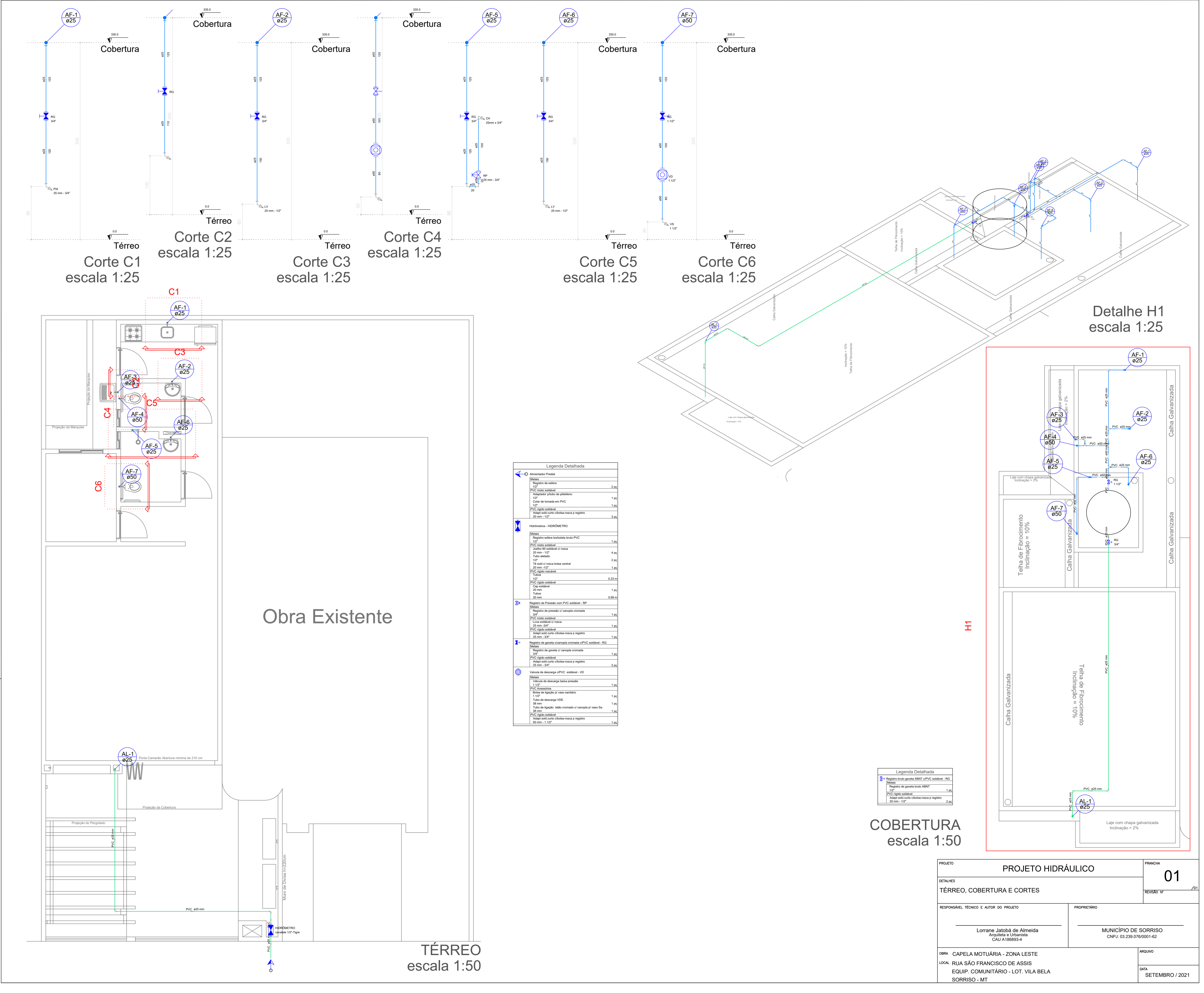
TÉRREO escala 1:50
