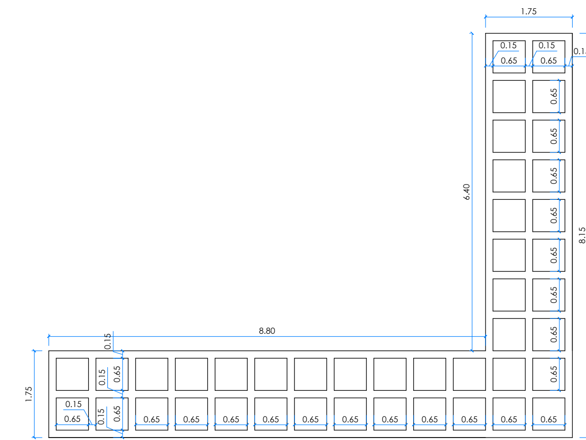
Detalhe do Pergolado Metálico Esc.: 1/75
