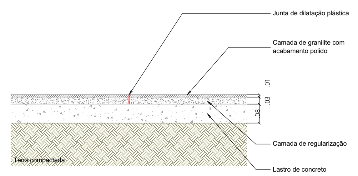
DET Piso Granilite 1:10
