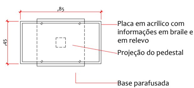
VISTA SUPERIOR DA BASE DO MAPA TÁTIL ESCALA: 1/25
