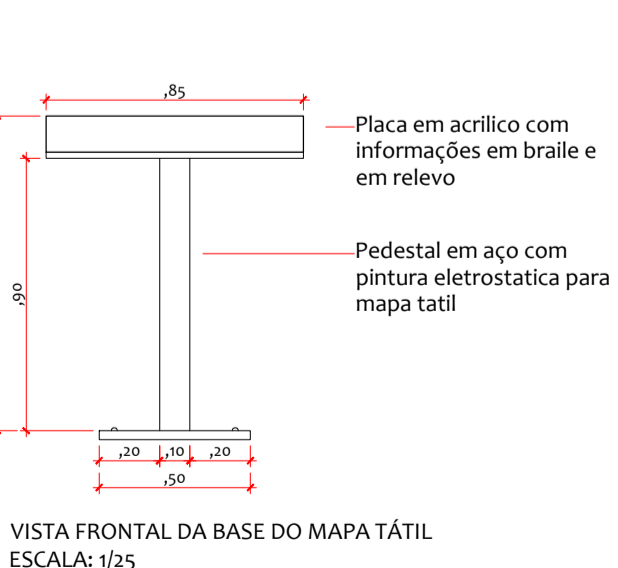
VISTA FRONTAL DA BASE DO MAPA TÁTIL ESCALA: 1/25
