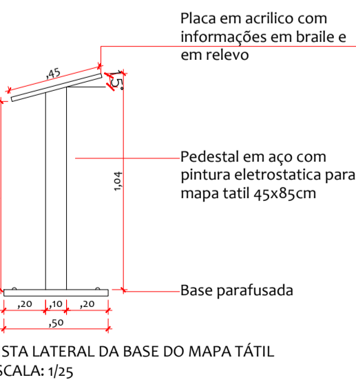
VISTA LATERAL DA BASE DO MAPA TÁTIL ESCALA: 1/25
