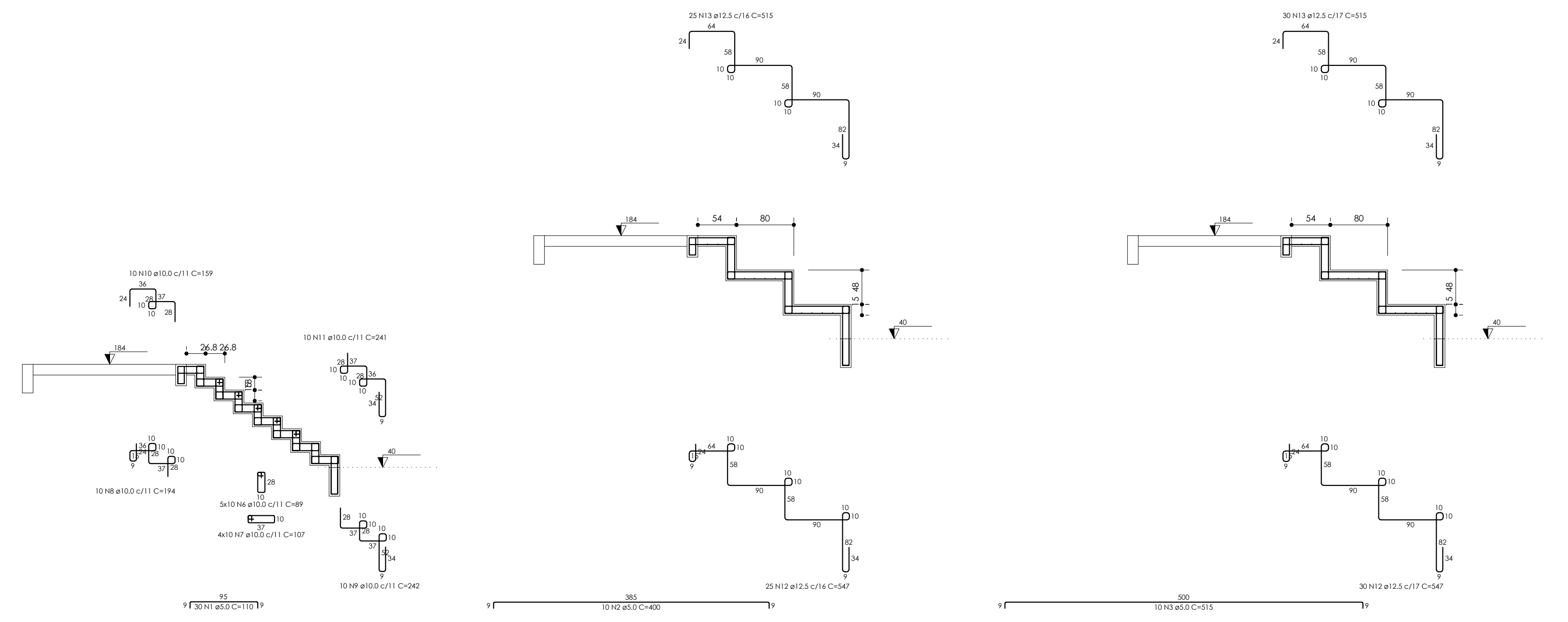
Corte A-A (LE1) ESC: 1/30
