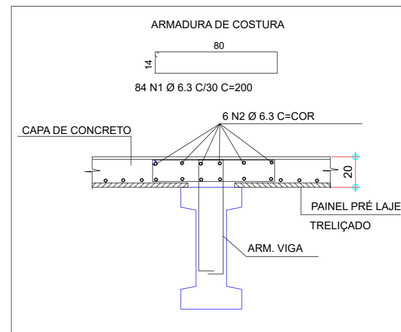
VISTA TRANSVERSAL - DETALHE REGIÃO DE APOIO NA LAJE Escala / 1:50
