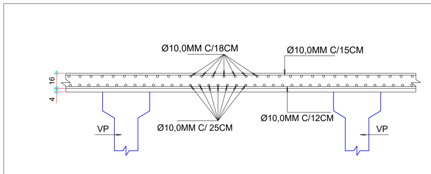
VISTA TRANSVERSAL - ARMADURA DE LAJE Escala / 1:50
