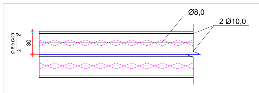
VISTA SUPERIOR - DETALHE VIGOTAS PRÉ LAJE Escala / 1:25
