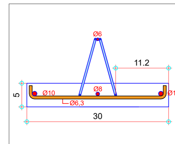
VISTA TRANSVERSAL - DETALHE VIGOTAS PRÉ LAJE Escala / 1:5
