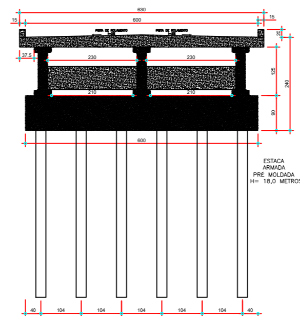
VISTA TRANSVERSAL - PONTE
