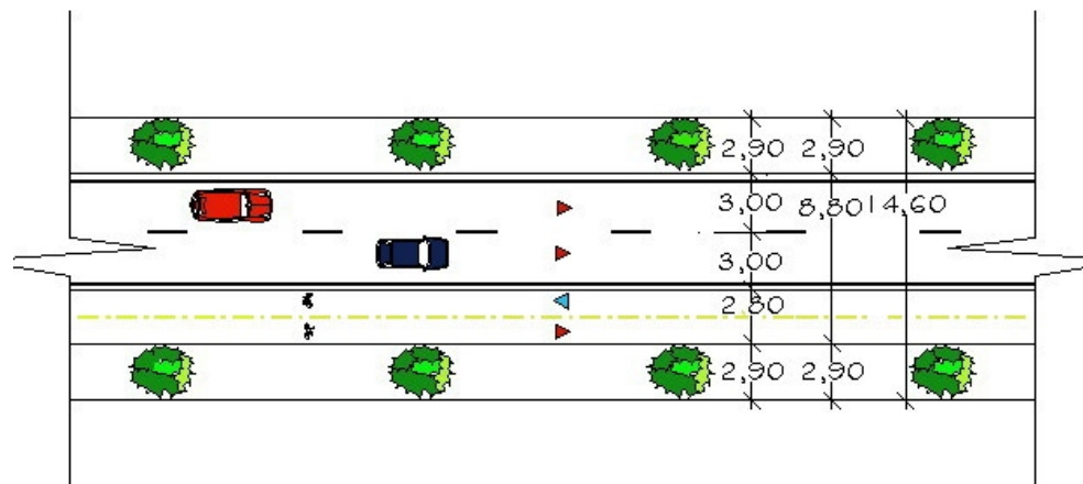
PLANTA BAIXA - Rua Lupicínio Rodrigues
