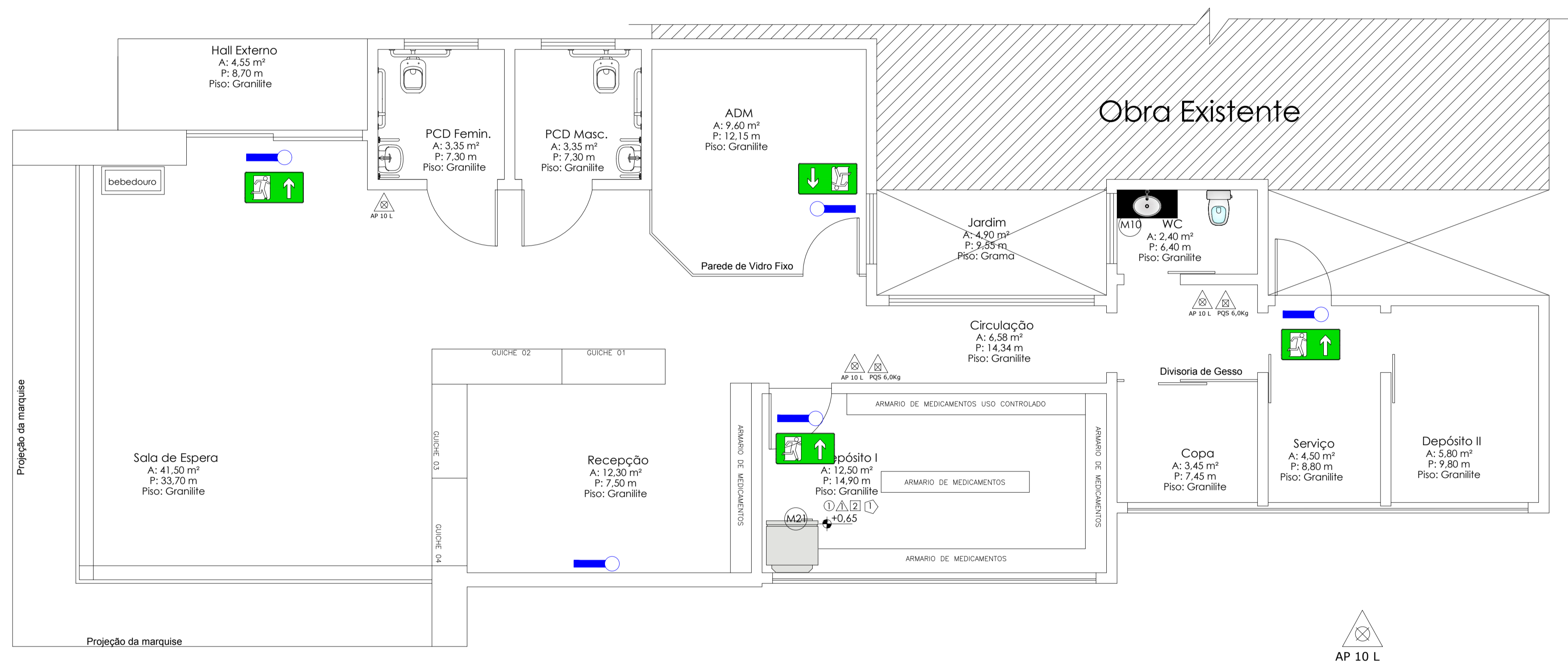
5 Planta de Incêndio Esc.: 1/50
