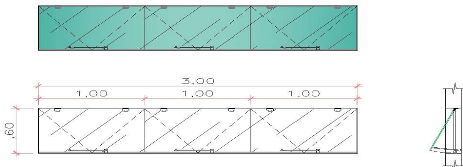
Figura 1: Corte e vista da janela (3,00X0,80m).
