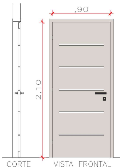
Figura 1: Vista frontal e Corte da porta metálica de (0,90x2,10m).
