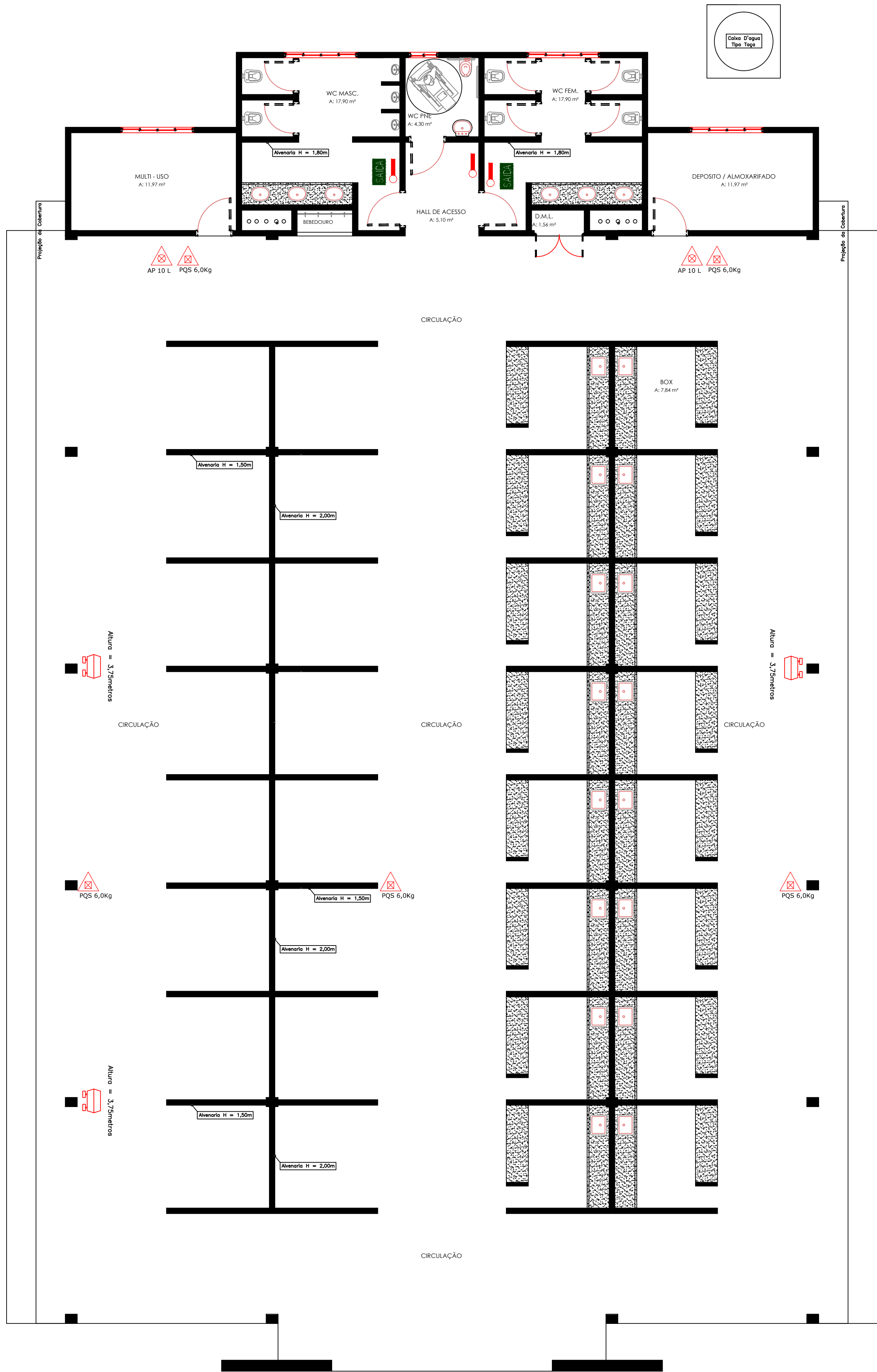
Planta Baixa Esc.: 1/75
