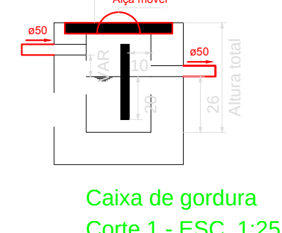
Caixa de gordura
