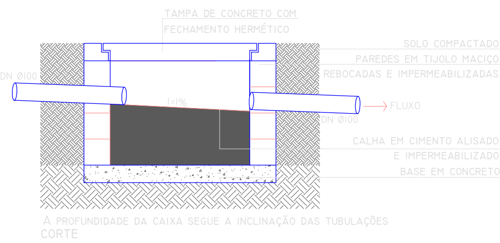
CAIXA DE INSPEÇÃO ESGOTO 60x60cm
