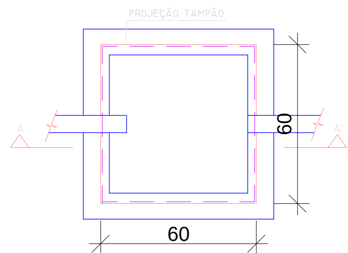
CAIXA DE INSPEÇÃO ESGOTO 60x60cm
