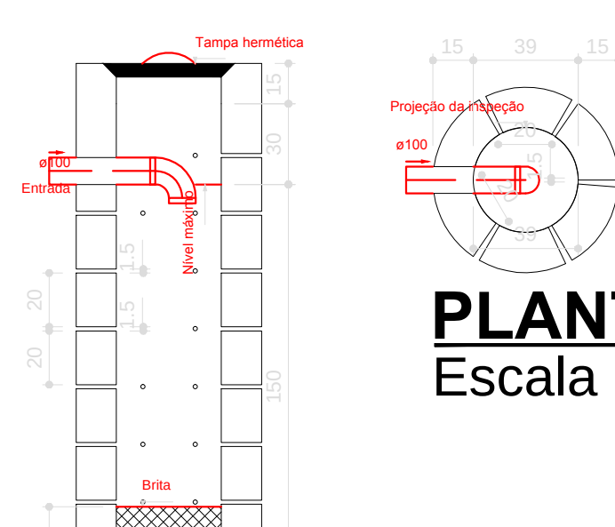
Caixa de gordura
