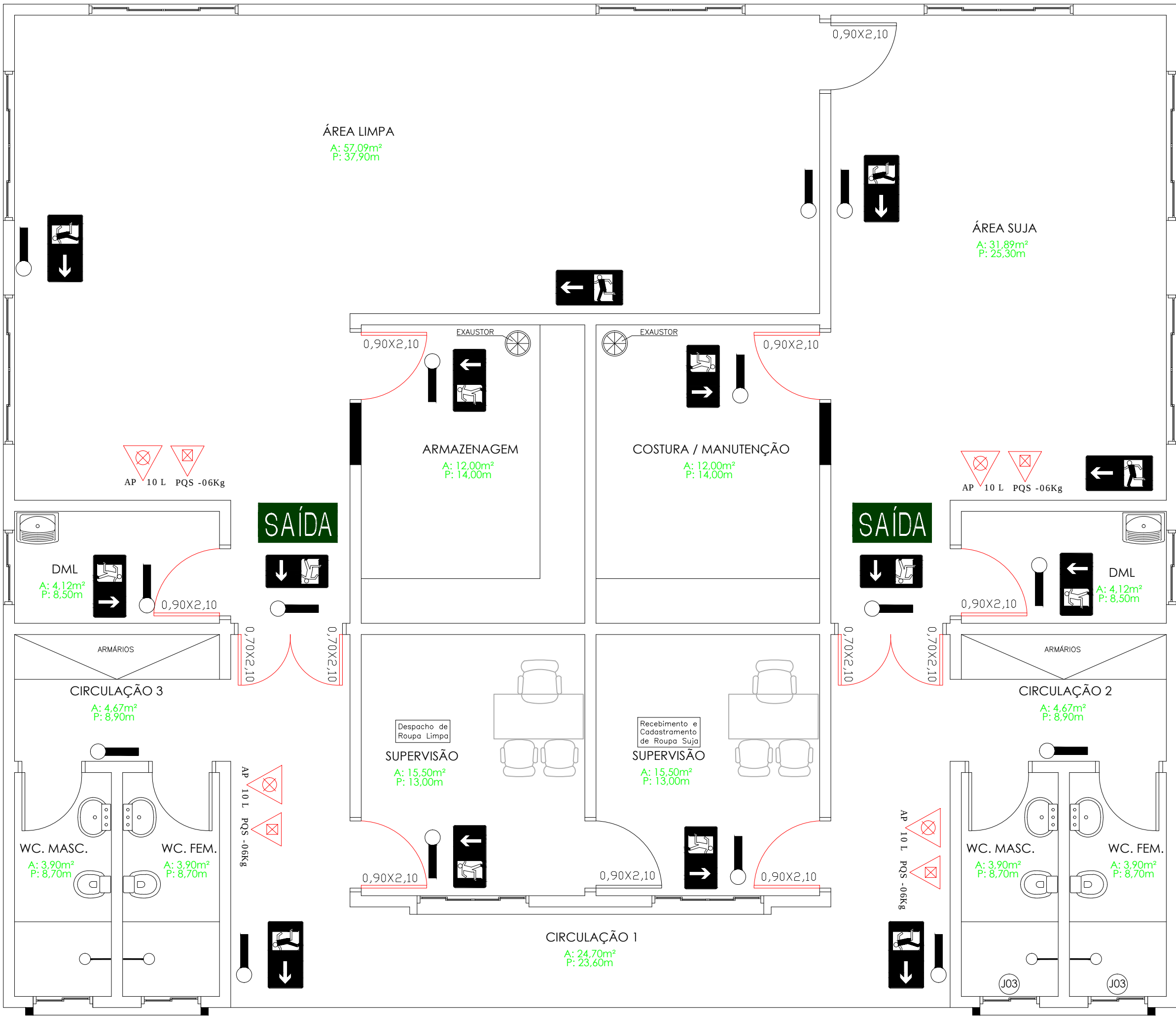
Planta Baixa - LAVANDERIA Esc.: 1/75
