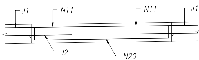
DETALHE 1 ESCALA 1:25
